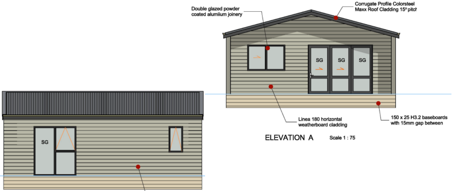
ELEVATION B
